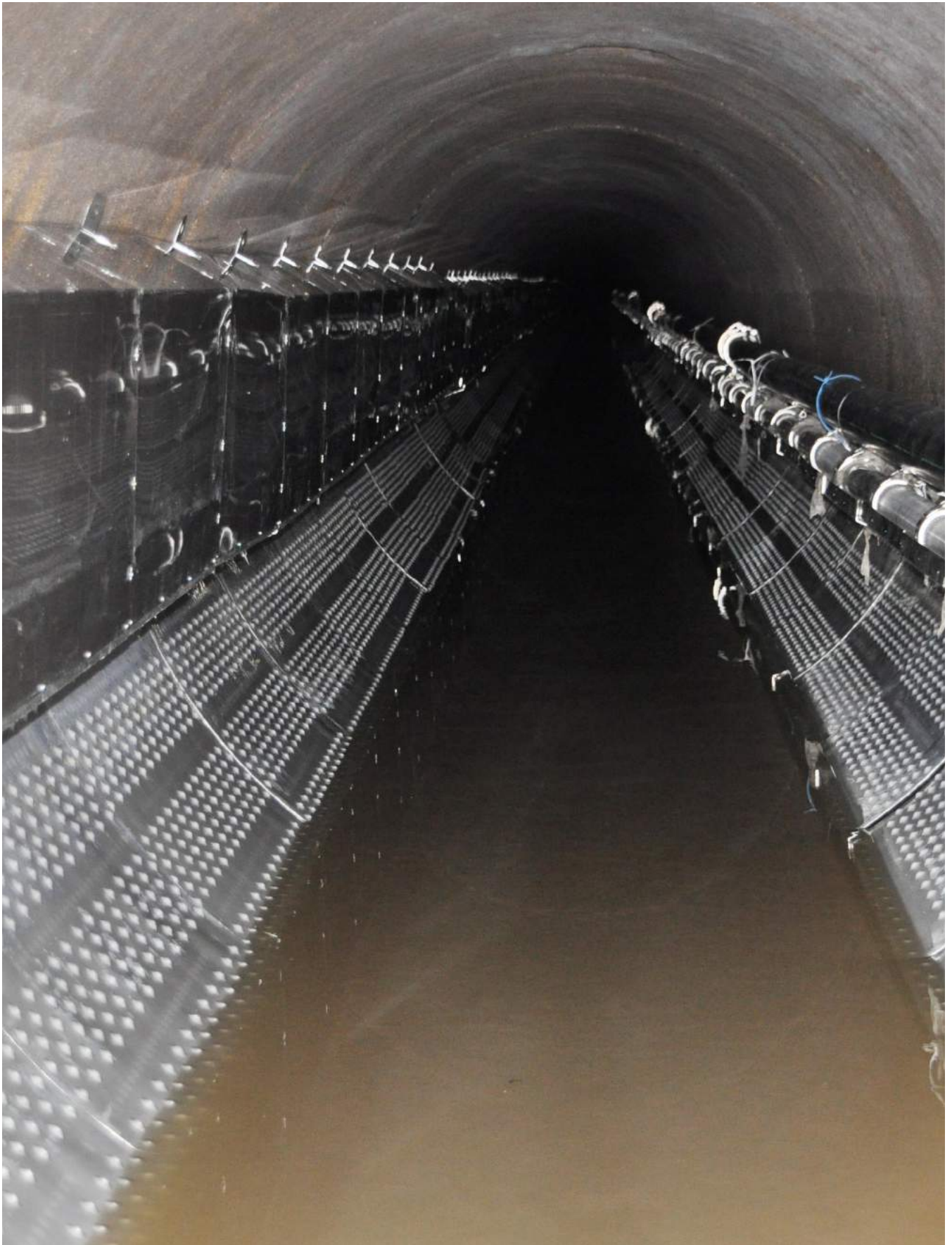
Abwasserwärmeprojekt des OÖWW am Alten Stadthafen: Blick in den Mischwasserkanal mit einem Durchmesser von 1,50 Meter. (Die Installation der Wärmetauscher ist noch nicht abgeschlossen.)
