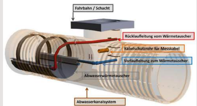
Systemskizze: OOWV-Pilotprojekt zur Nutzung von Abwasserwärme
